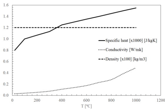
c) Rockwool
